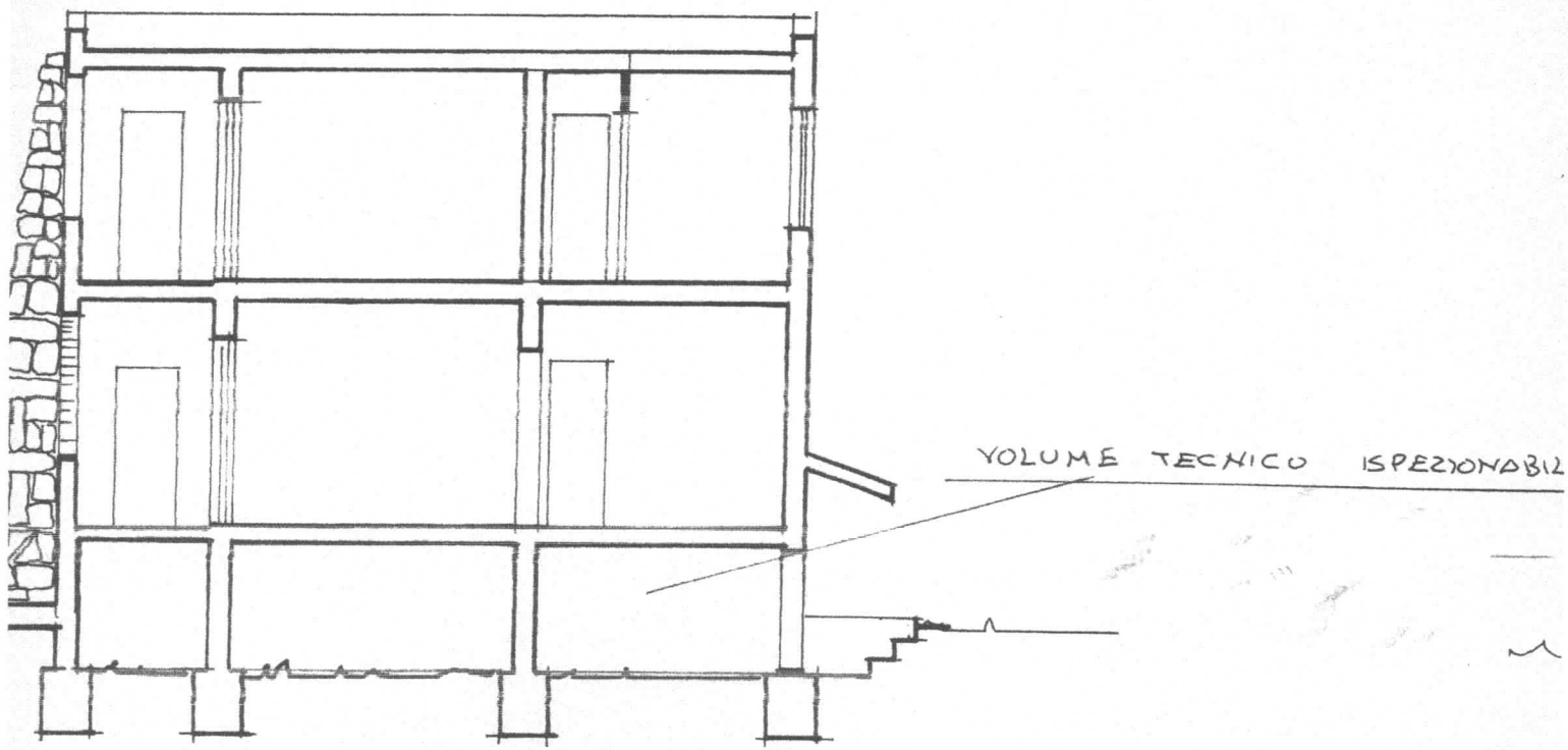
SEZIONE ΔΔ 1:100
